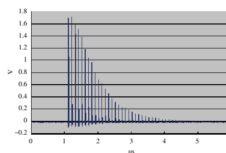
図4 長光路化したCRDS波形
