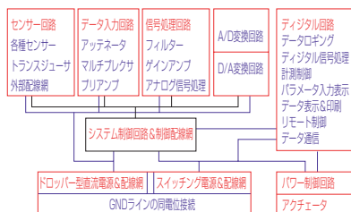
図1 共通するアナログ回路の回路構成
